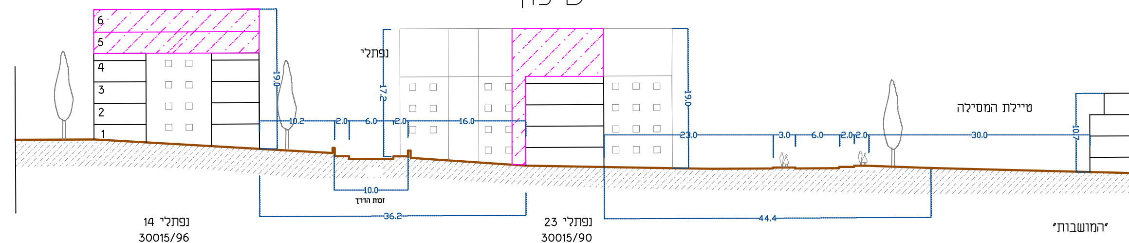
ה-ה חתך דרך רחוב גד-מוצע
