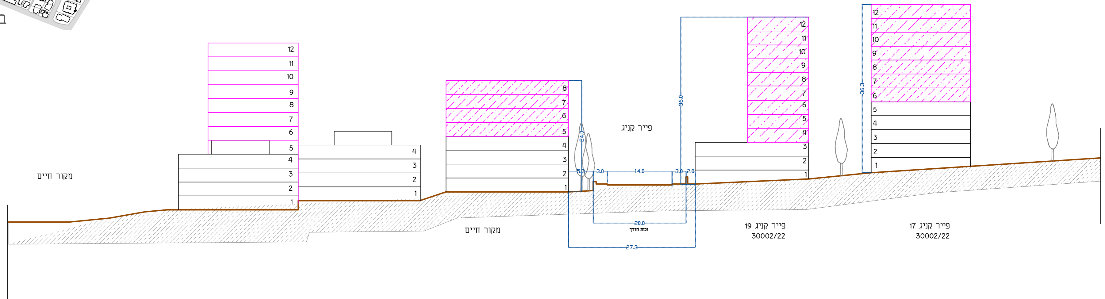
ג-ג חתך דרך רחוב פייר קניג-מוצע
